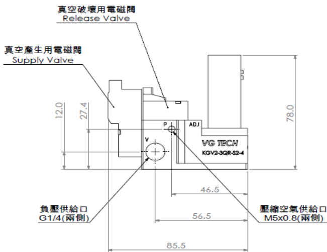
KGV2連座底座尺寸表(mm)
