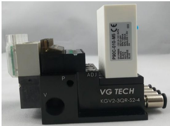
四連座負壓切換模組產品照片
